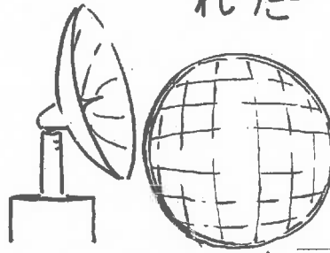
れーざー
