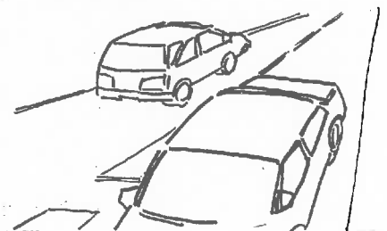
どうろ
