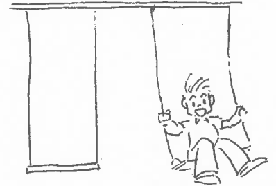
ぶらんこ
